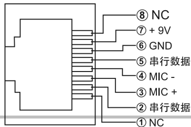
◇ 麦克风连接头示意图 (连接头的前视图)
